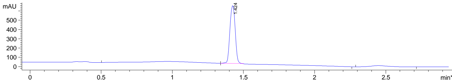
*DAD1 B, Sig=254,16 Ref=360,100
